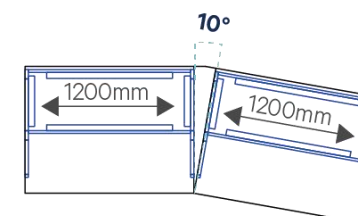
10° Console
